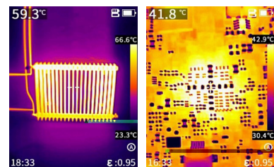
PCBA
